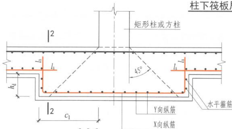
柱下筏板局部增加板厚构造(二)
