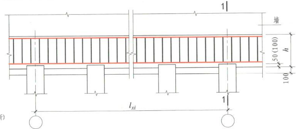
墙下单排桩承台梁CTL钢筋构造
