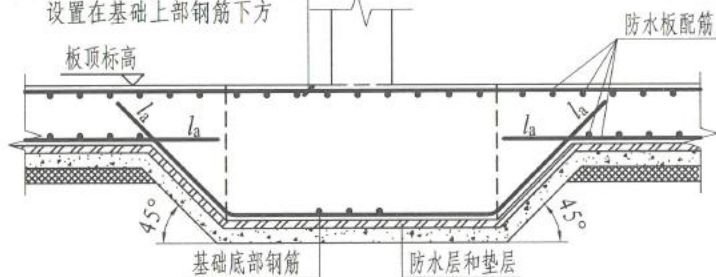
高板位防水底板
