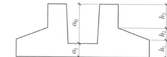
图2.3.2-8 锥形截面杯口独立基础竖向尺寸
