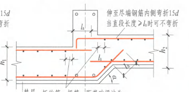
板的第一根筋,距基础梁边为1/2板筋间距,且不大于75mm (b) 板顶、板底均有高差
