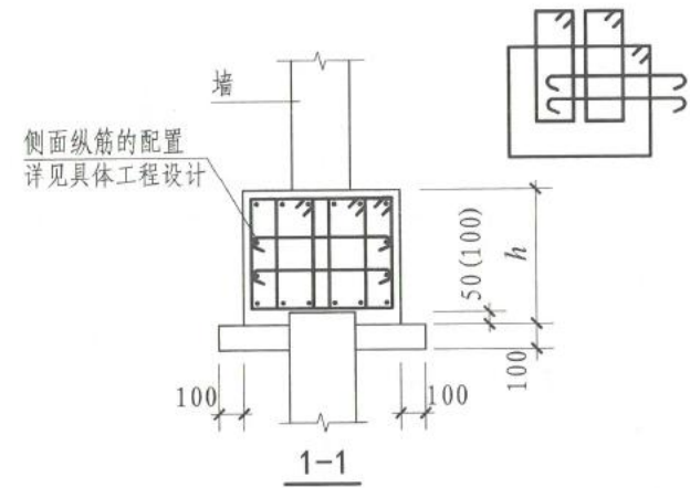
墙下单排桩承台梁CTL钢筋构造
