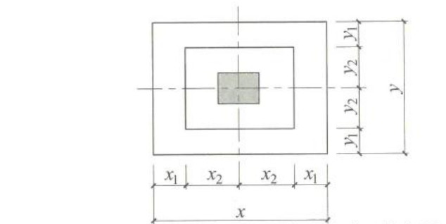
图2.3.3-1 对称阶形截面普通独立基础原位标注
