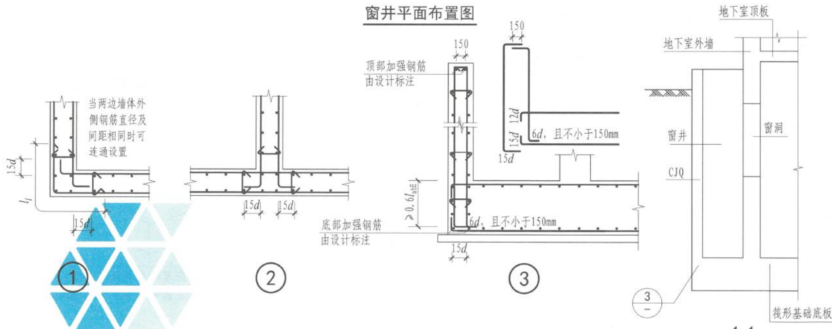
窗井墙CJQ配筋构造
