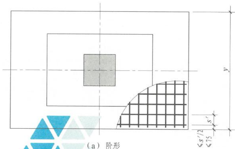
独立基础DJj、DJz、BJj、BJz底板配筋构造
