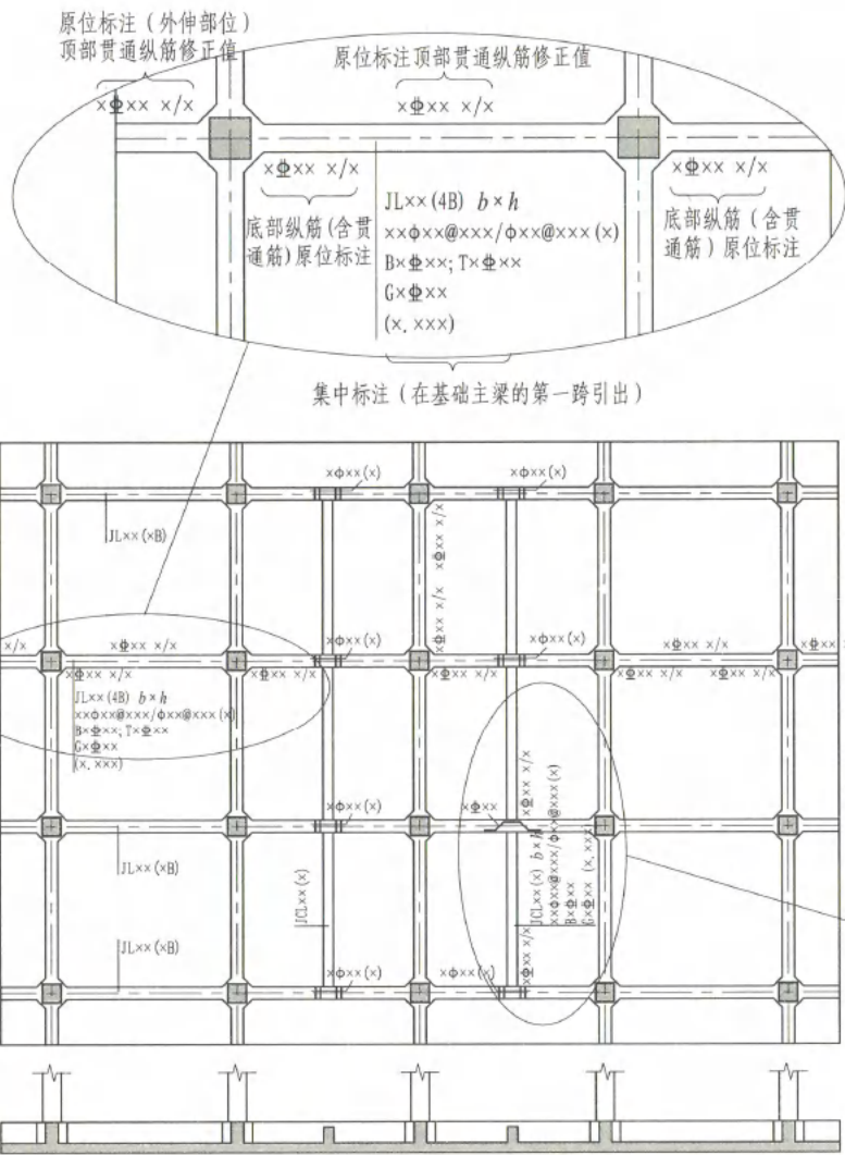
1-1 基础主梁JL与基础次梁JCL标注图示
