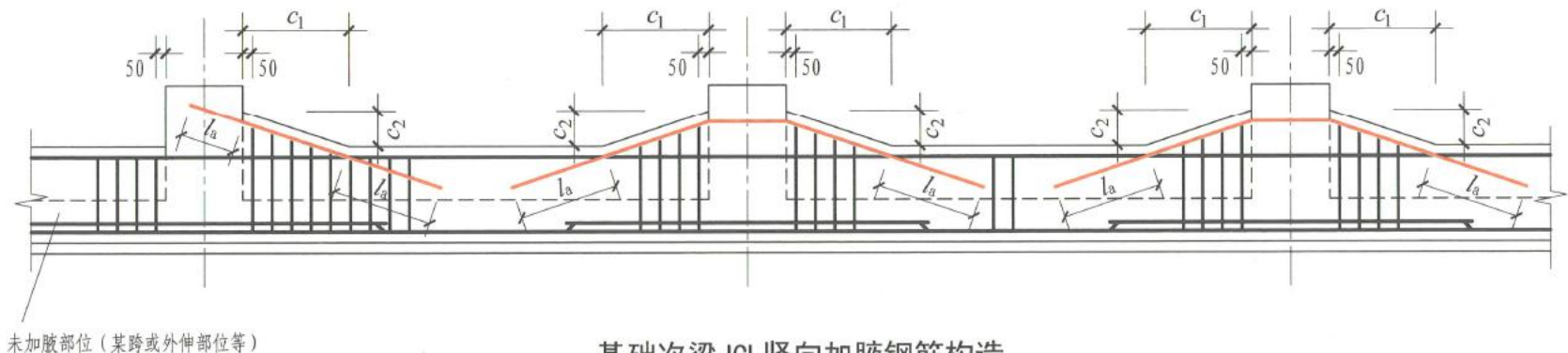
基础次梁JCL竖向加腋钢筋构造
