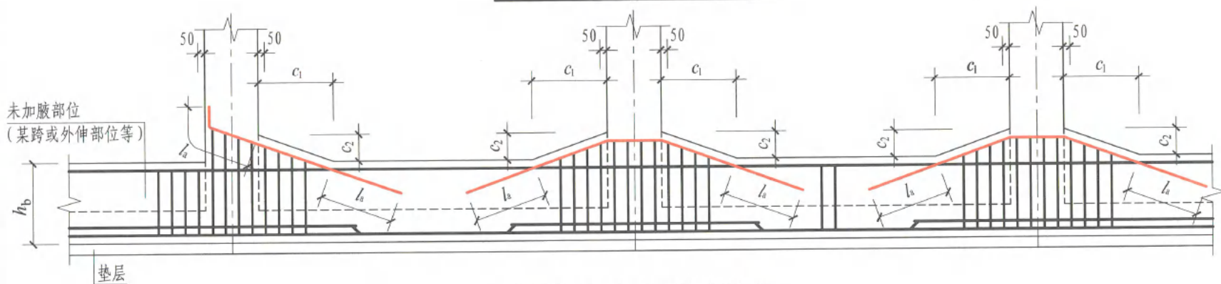
基础梁JL竖向加腋钢筋构造
