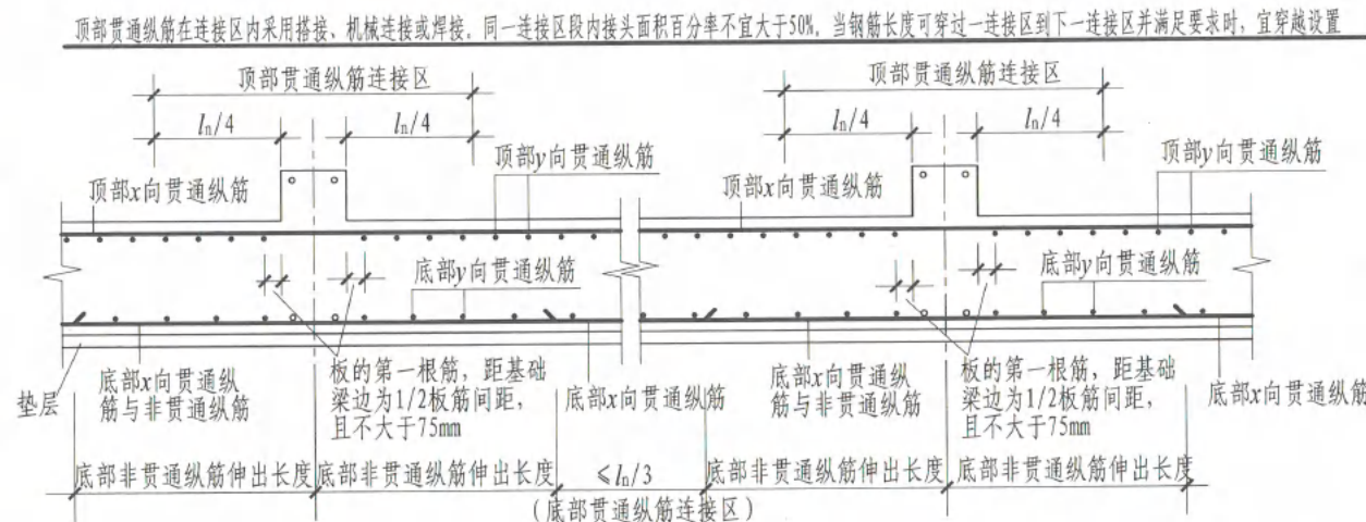
梁板式筏形基础平板LPB钢筋构造
