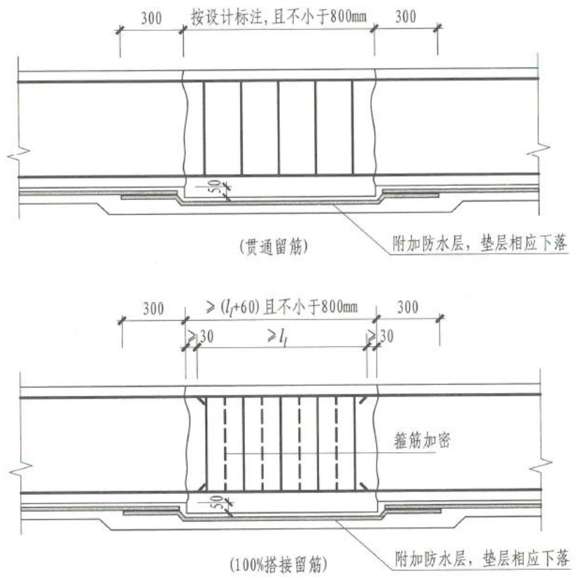
基础梁后浇带HJD构造
