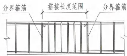
梁、柱类构件纵向受力钢筋搭接接头区箍筋构造
