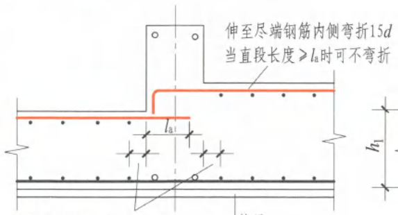
板的第一根筋,距基础梁边为1/2板筋间距,且不大于75mm (a) 板顶有高差
