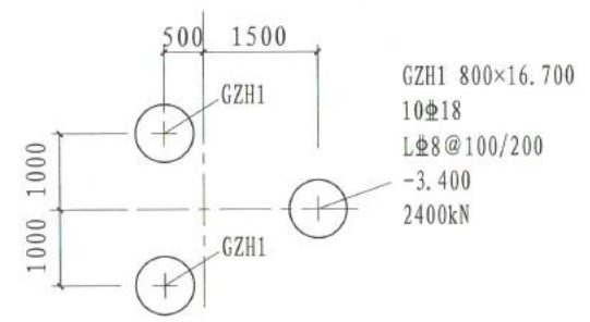
图6.2.1 灌注桩平面注写示意
