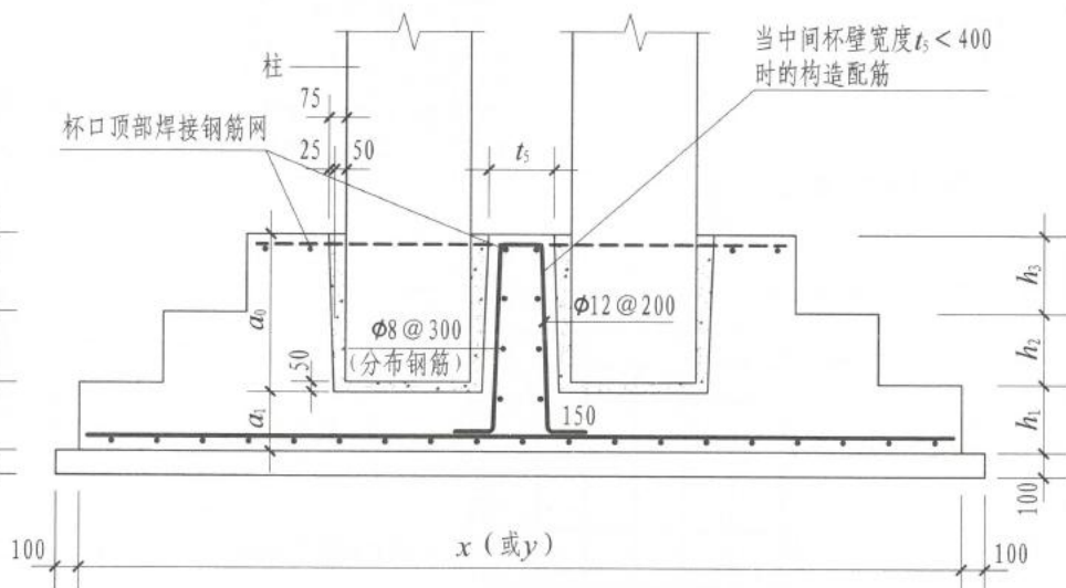
双杯口独立基础构造
