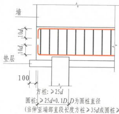
承台梁端部钢筋构造
