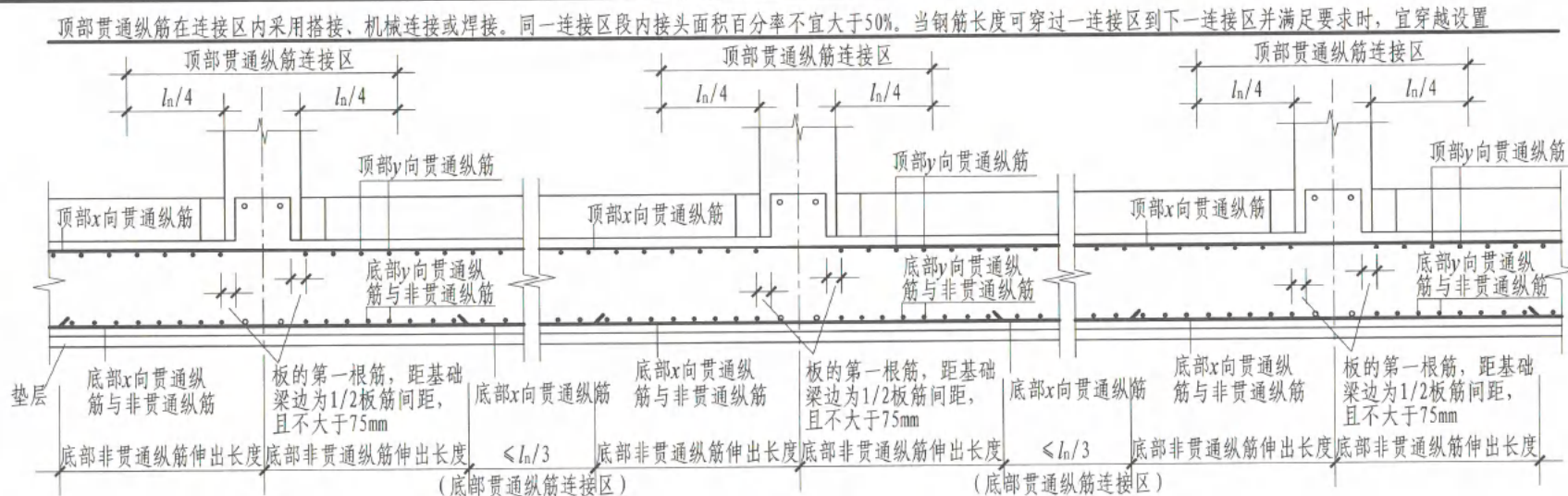
梁板式筏形基础平板LPB钢筋构造 (柱下区域)
