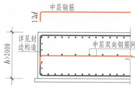
中层筋端头构造
