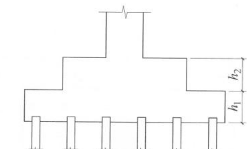
图6.6.2-1 阶形截面独立承台竖向尺寸
