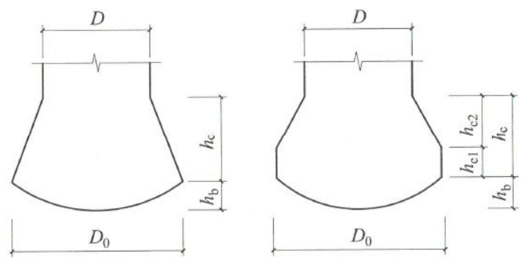
图6.2.2 扩底灌注桩扩底端示意
