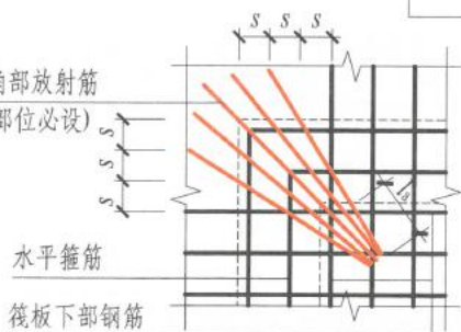
柱下筏板局部增加板厚角部放射筋
