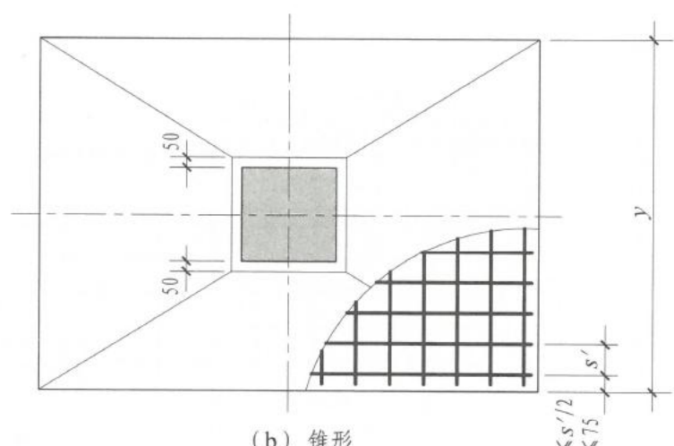
独立基础DJj、DJz、BJj、BJz底板配筋构造
