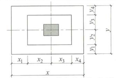
图2.3.3-2 非对称阶形截面普通独立基础原位标注
