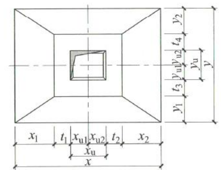
图2.3.3-8 锥形截面杯口独立基础原位标注(一)
