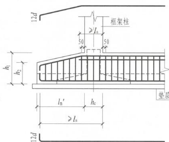
条形基础梁端部变截面外伸构造
