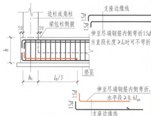
梁板式筏形基础梁端部无外伸构造
