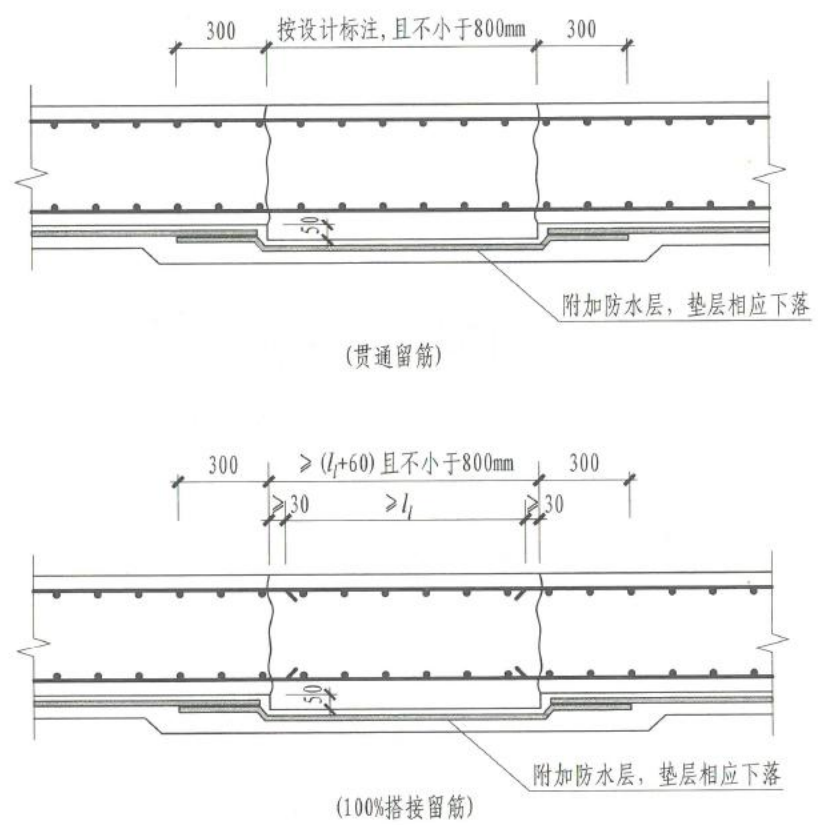
基础底板后浇带HJD构造
