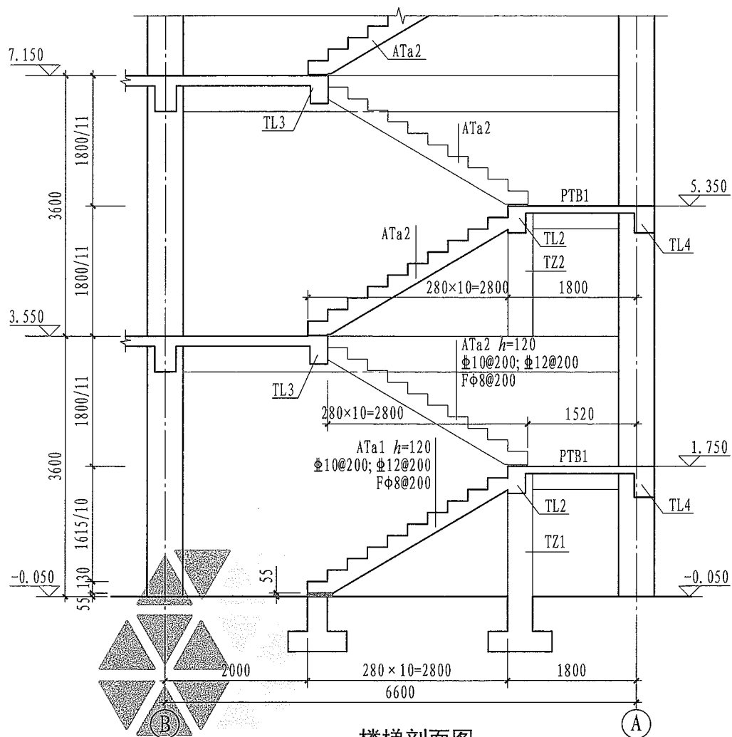
楼梯剖面图
