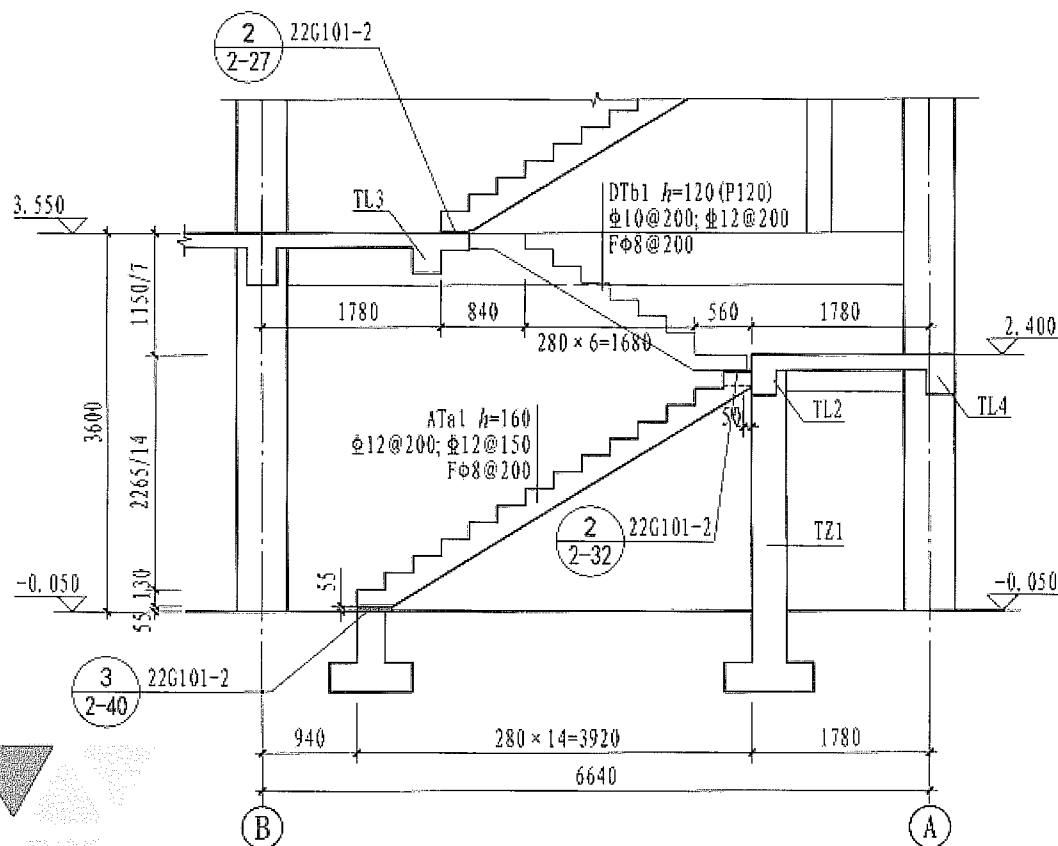
楼梯剖面图 (局部示意)
