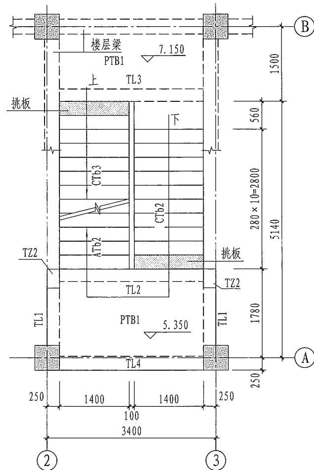
▽5.350~▽7.150楼梯平面图
