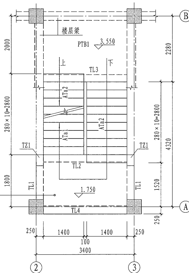
▽1.750~▽3.550楼梯平面图
