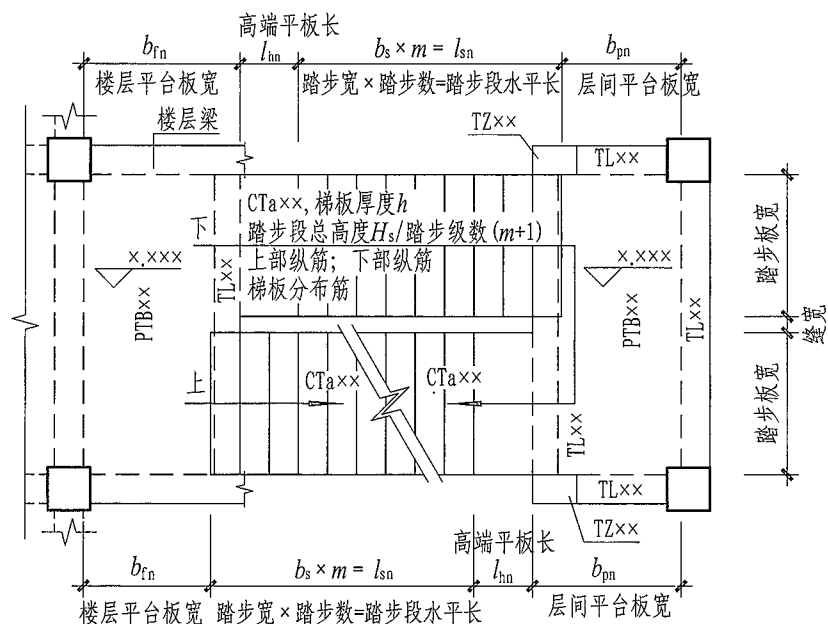
图1 \nabla x. xxx ~ \nabla x. xxx 楼梯平面图 (CTa型注写方式)
