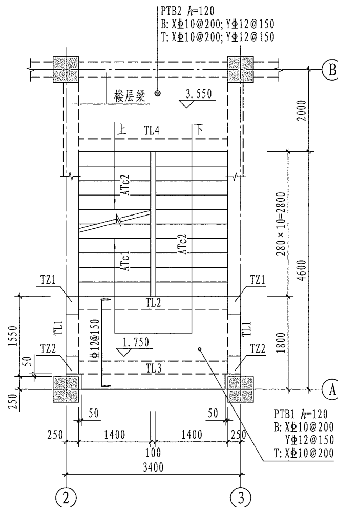
▽1.750~▽3.550楼梯平面图
