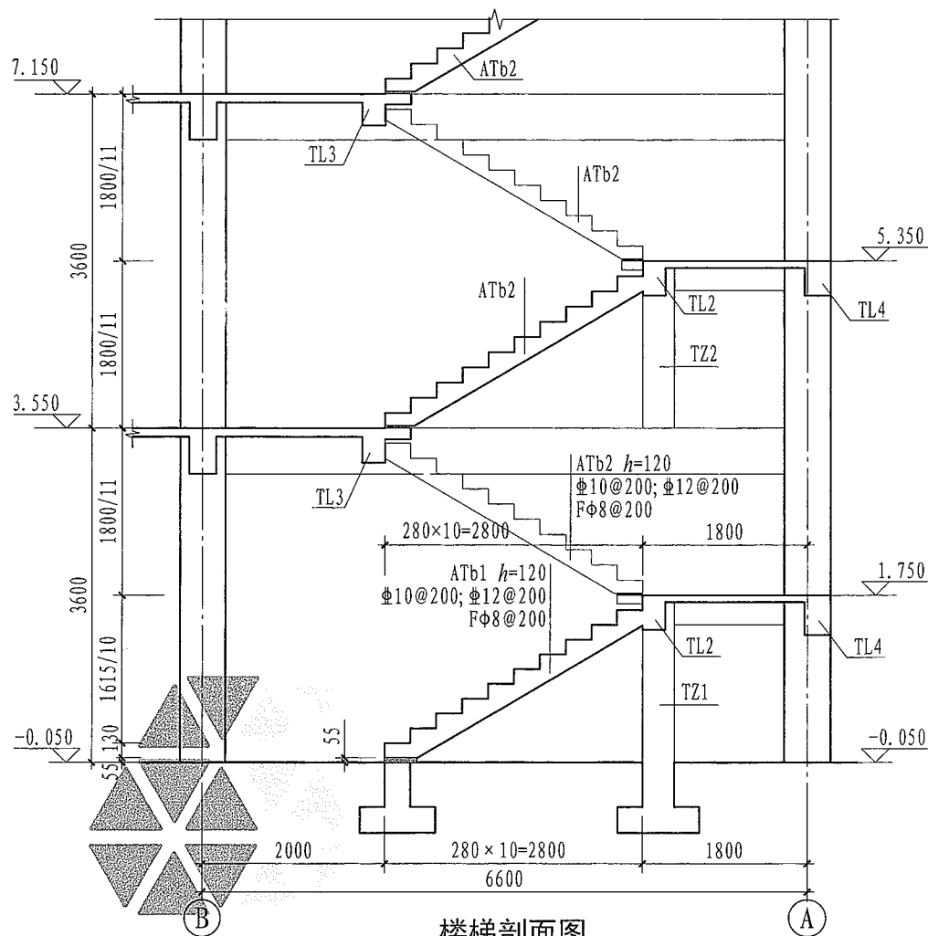
楼梯剖面图
