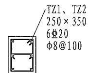
TZ1、TZ2
